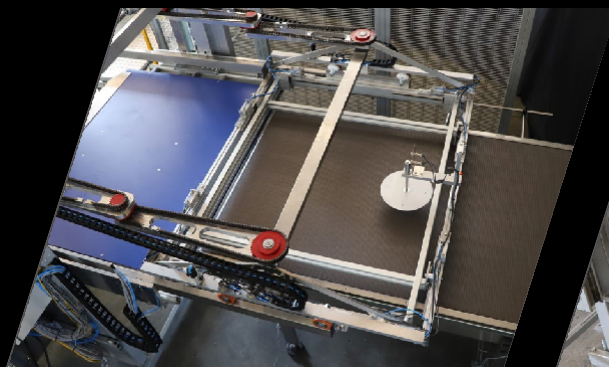
-Testata di trasferimento a spinta delle bottiglie sul banco -Cabeçote de transferência de garrafas para o banco de acumulação
