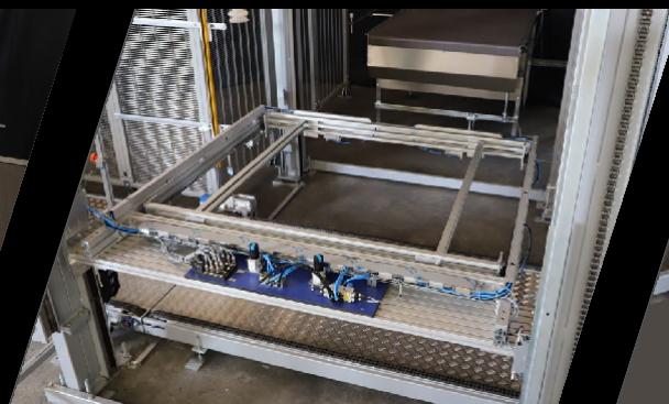
-Centratore perimetrale indipendente per compattare lo strato -Centrador perimetral independente para compactar o estrato
