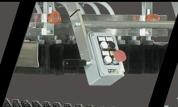
-Pulsantiera sulla testata alto-basso presa rilascio bottiglie -Painel de controlo de carga e de descarga das garrafas
