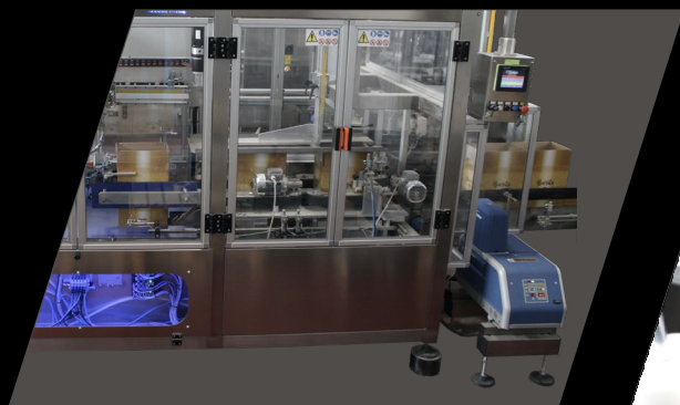
-Chiusura inferiore del cartone con colla -Fecho do fundo da caixa com cola
