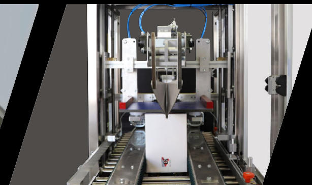
-Chiusura delle falde superiori con flap -Sistema flap para fecho das abas superiores
