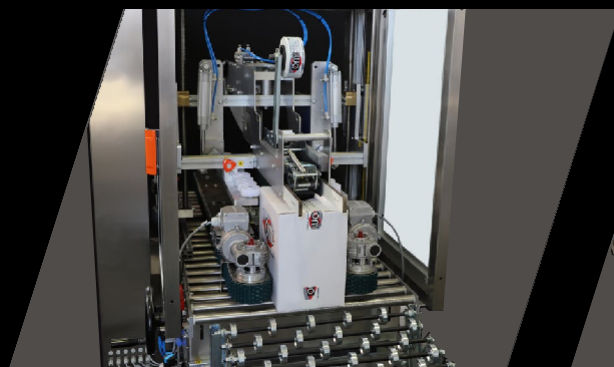
-Chiusura del cartone con nastro adesivo -Fecho de caixa - fita adesiva
