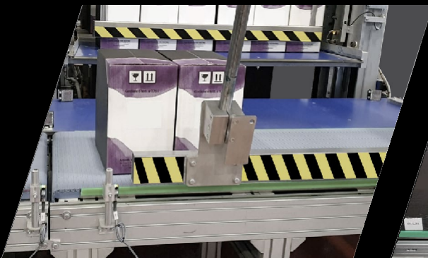
-Millennium 3.000 Evo HS con doppio braccio spintore fino a 2.000 c/h Patented -Millennium 3.000 Evo HS com braço empurador duplo produção até 2.000 cx/h Patenteado
