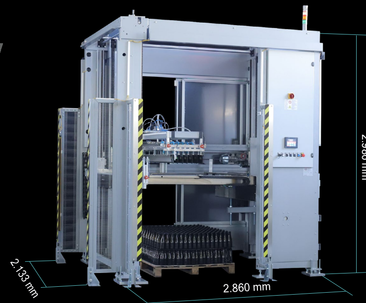
-Centratore perimetrale per compattare lo strato -Centrador perimetral para compactação do estrato
